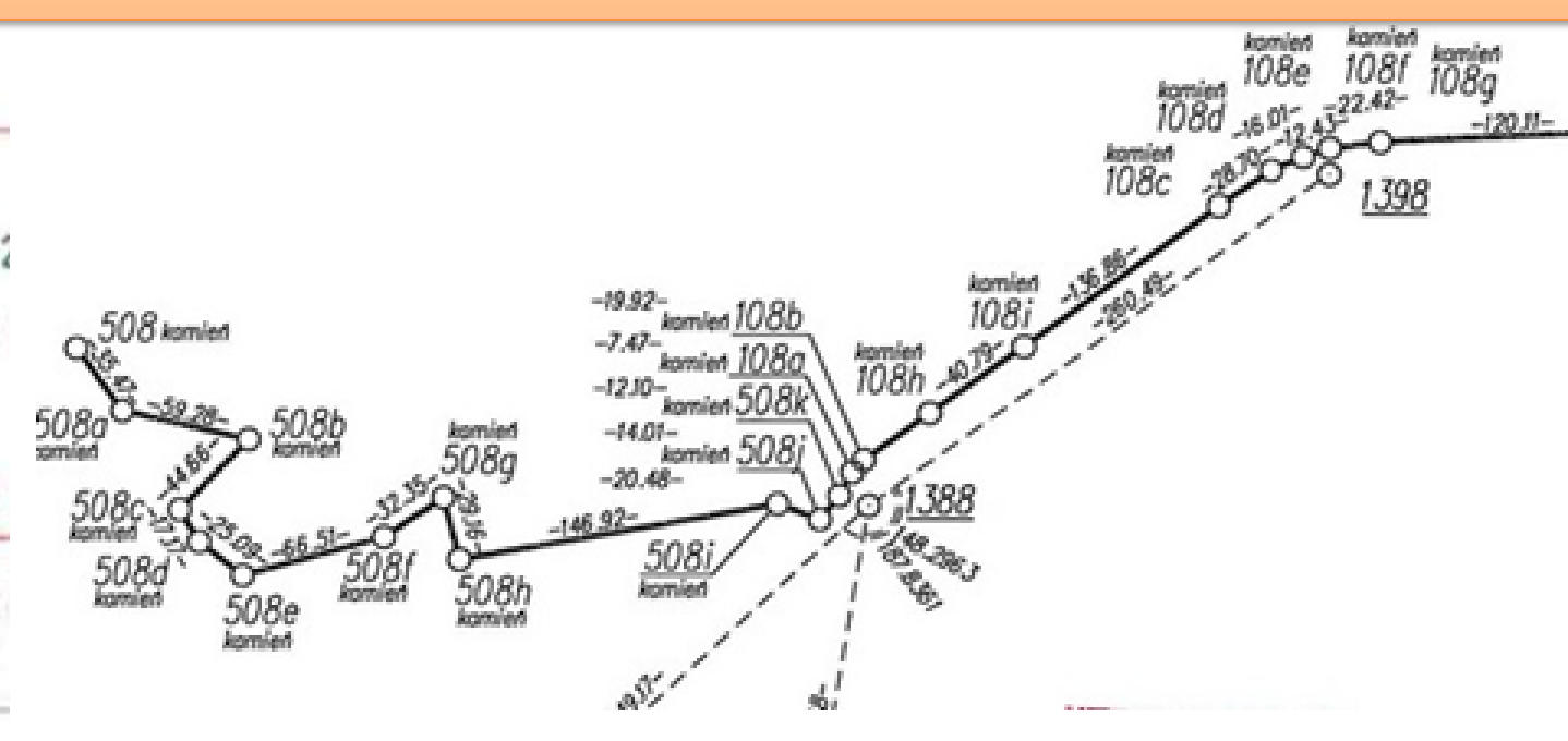
Rysunek 2. Fragment szkicu ustalenia i pomiaru punktów granic Źródło: WBGiTR Częstochowa, PODGiK Zawiercie
